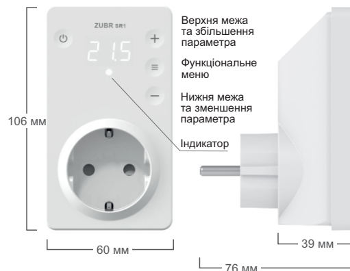
Рисунок 1. Габаритні розміри SR1
